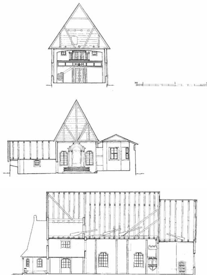
Uppmätningsritningar ur Medeltida träkyrkor del I . G Wirén 1978.
